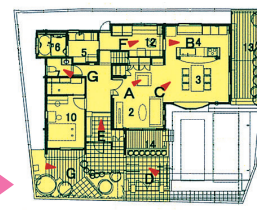
配置図兼1階平面図
