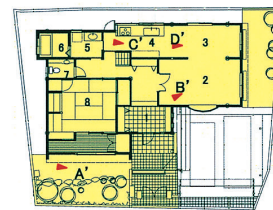
配置図兼1階平面図
